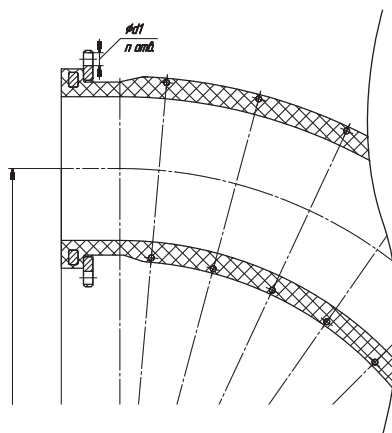
Закладной фланец
