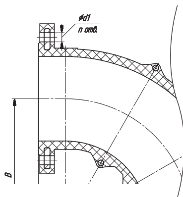
Закладной фланец
