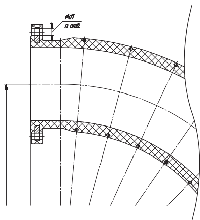
Закладной фланец
